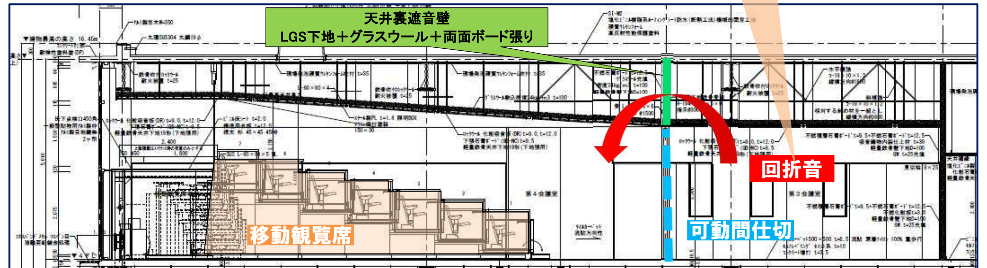
【 講堂 断面図 】
